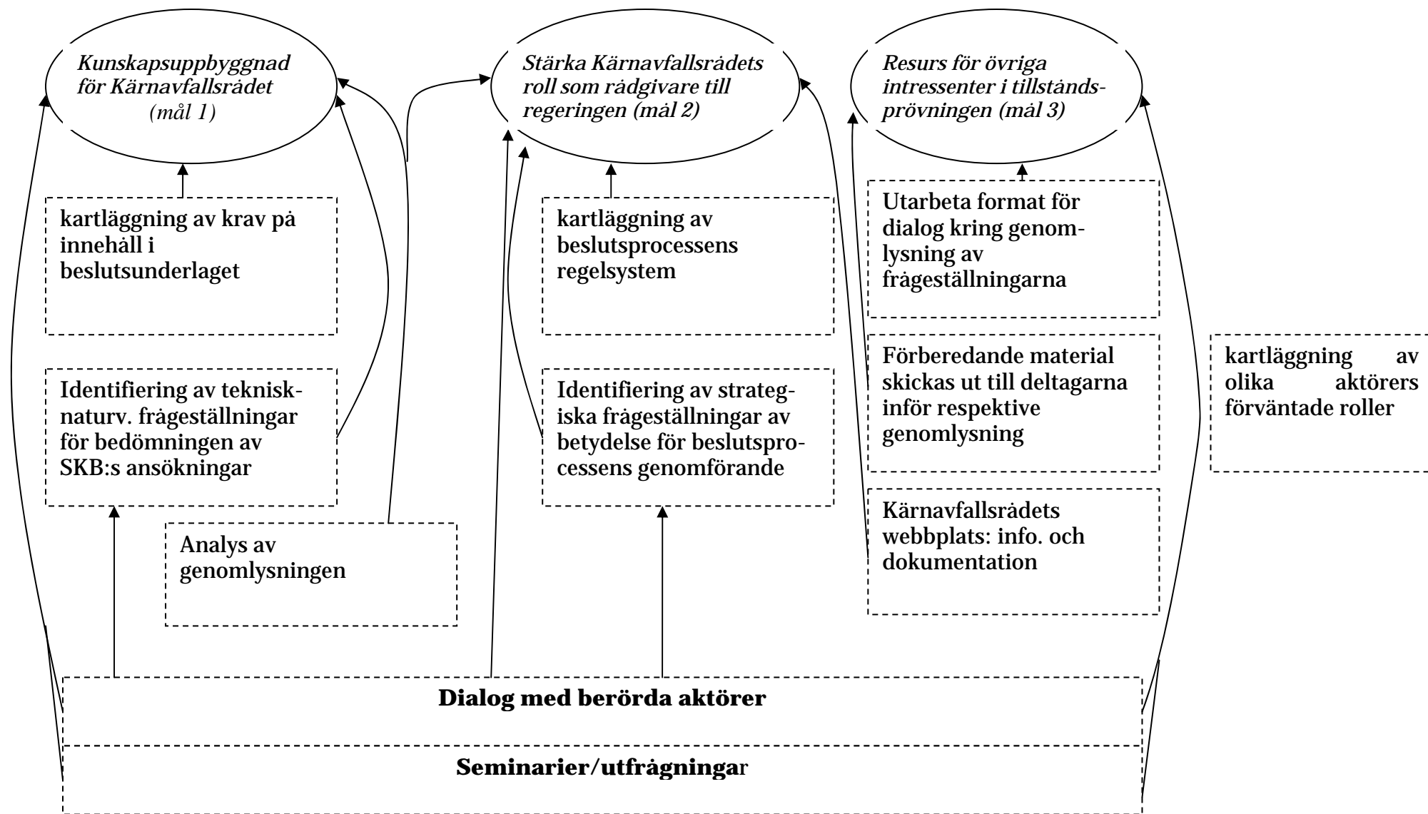
Figur 1. Genomlysningsprogrammets programlogik
